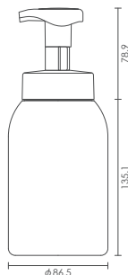
⑨ G3 600ml HDPE
